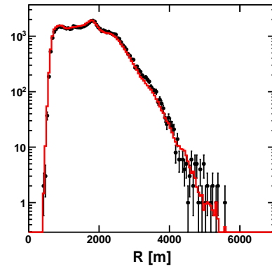
(d) Counter distance from the shower axis.
